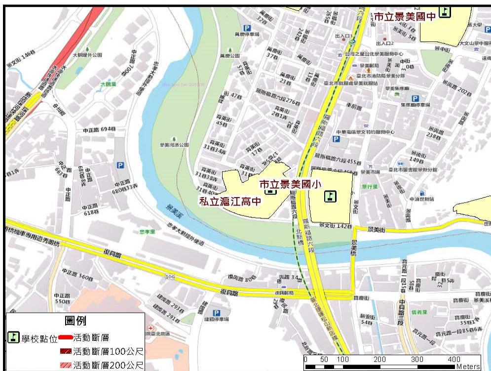
圖 2.4.1 地震災害潛勢圖 (瀏覽日期： 111 年 11 月 01 日)
