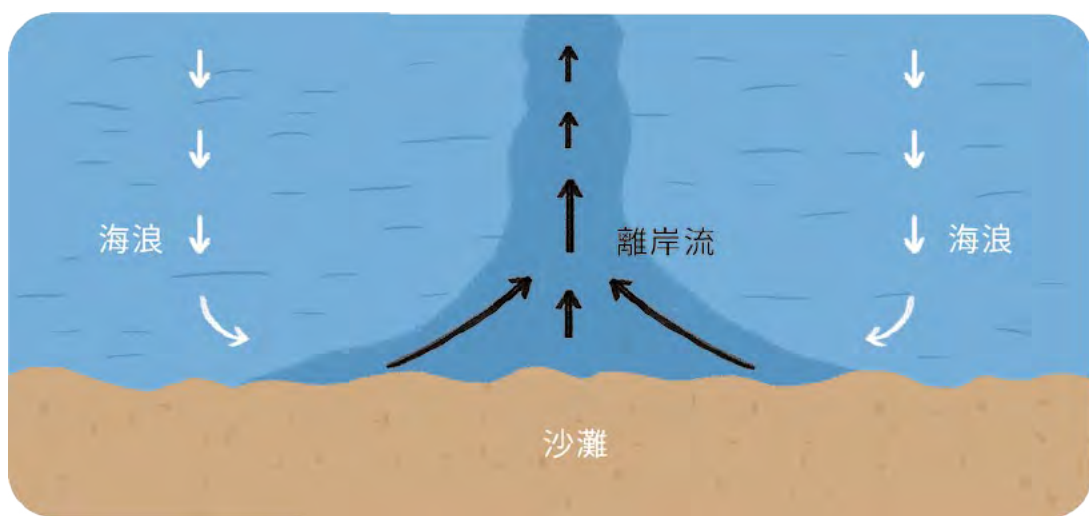
圖23. 離岸流形成示意圖
