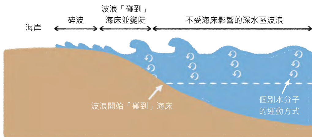
圖22. 海浪形成示意圖
