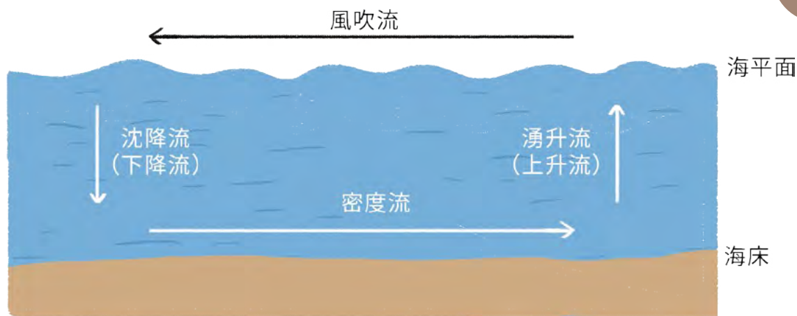
圖24. 洋流形成示意圖
